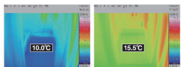
一般の断熱工法
